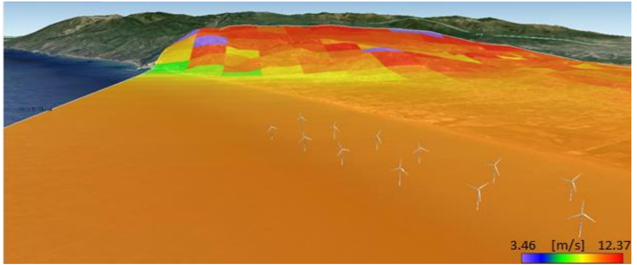
Şekil 6. Antakya körfezi olası türbin yerleşimi Google Earth izdüşümü ( Google Earth projection of probable wind turbine settlement at Antakya bay )
