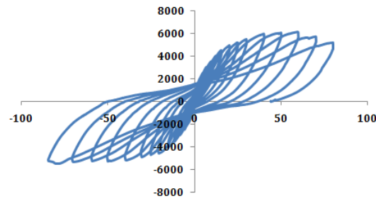
Şekil 11. S 2 Numunesinin Yük-Deplasman Grafiđi (Load-Displacementcurve of S 2 )
