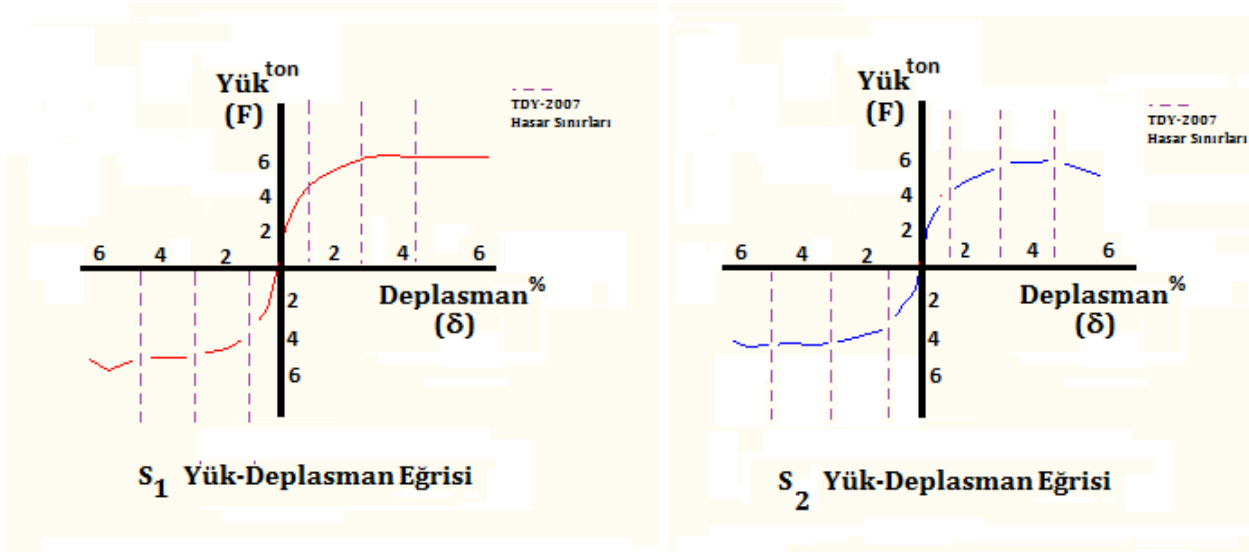
Şekil 13.S 1 Zarf Eğrisi (Capacity curve of S 1 )
