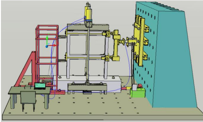
Şekil 5. Yükleme Düzenegi (Experimental setup)
