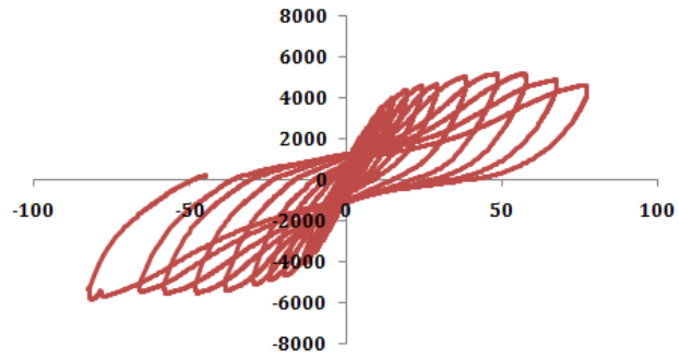
Şekil 12. S 3 Numunesinin Yük-Deplasman Grafiđi (Load-Displacementcurve of S 3 )
