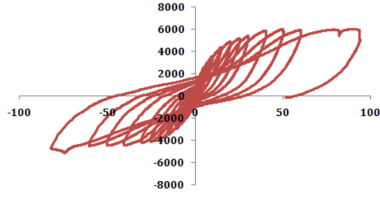
Şekil 10. S 1 numunesinin Yük-Deplasman Grafiđi (Load-Displacementcurve of S 1 )
