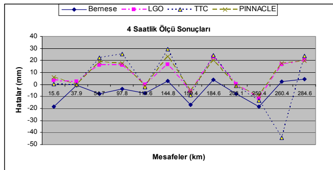
Şekil 9. 4 Saatlik Ölçü Sonuçları. Figure 9. 4 hours measurement results.
