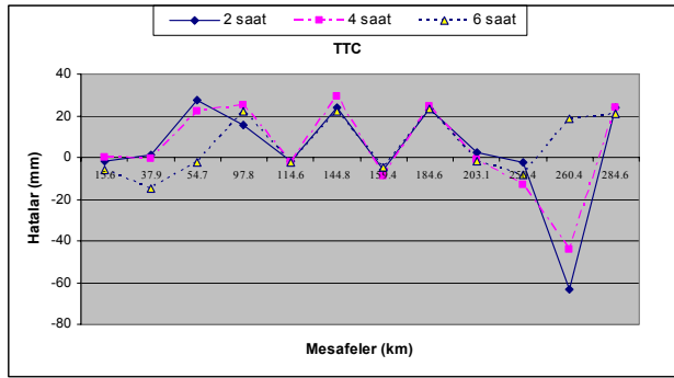
Şekil 6. TTC yazılımı ile elde edilen baz farkları. Figure 6. Baselines differences obtained using TTC software.
