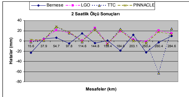
Şekil 8. 2 Saatlik Ölçü Sonuçları. Figure 8. 2 hours measurement results.
