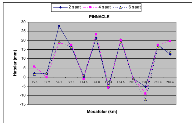
Şekil 7. PINNACLE yazılımı ile elde edilen baz farkları. Figure 7. Baselines differences obtained using Pinnacle software.
